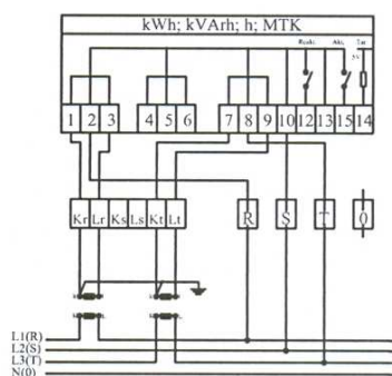
Dvosistemska poludirektna veza
