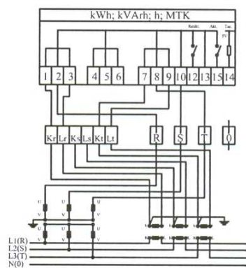
Trosistemska indirektna veza
