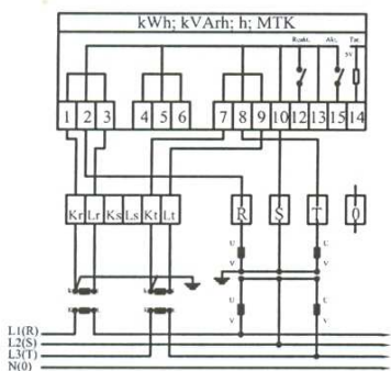
Dvosistemska indirektna veza
