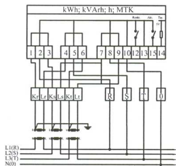
Trosistemska poludirektna veza
